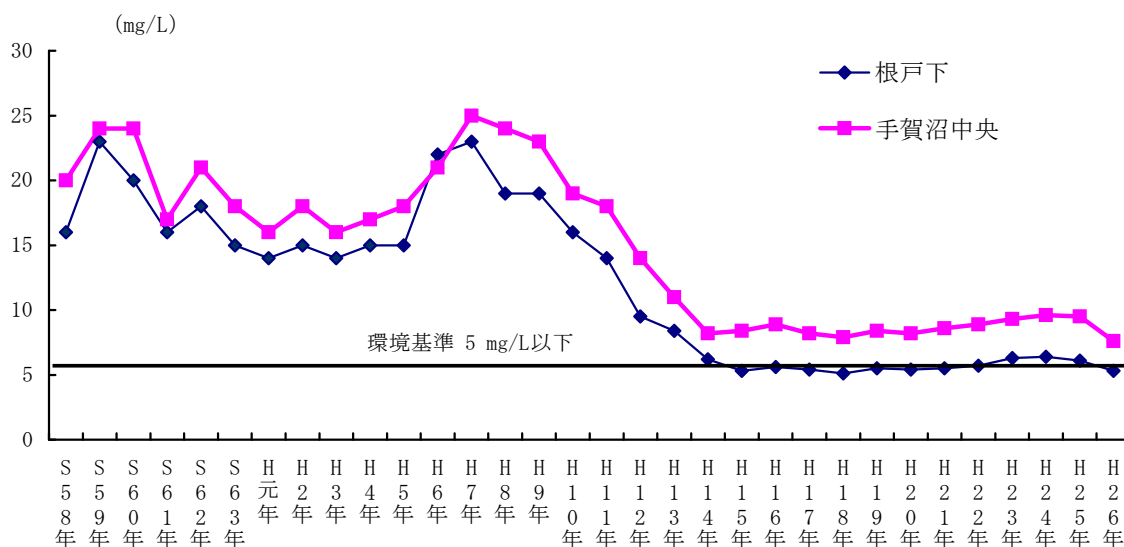
図1-5 手賀沼のCODの経年変化（年平均値）
