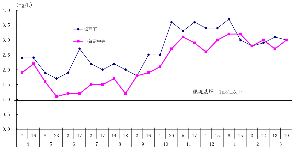
図1-9 手賀沼の全窒素の月別変化(平成26年度)
