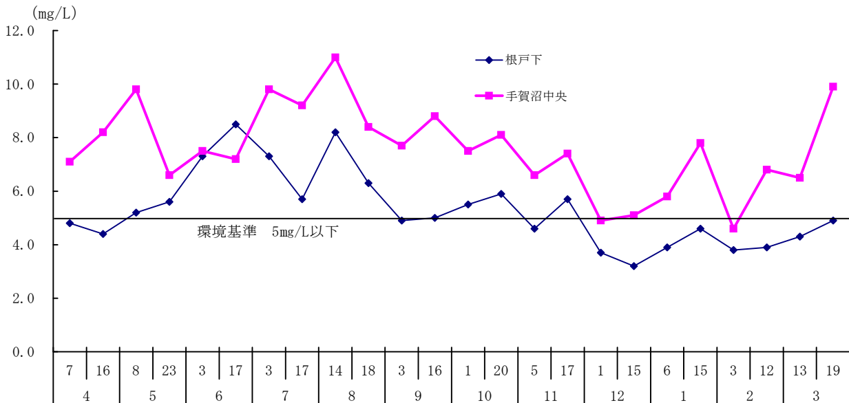
図 1-8 手賀沼のCODの月別変化 (平成26年度)
